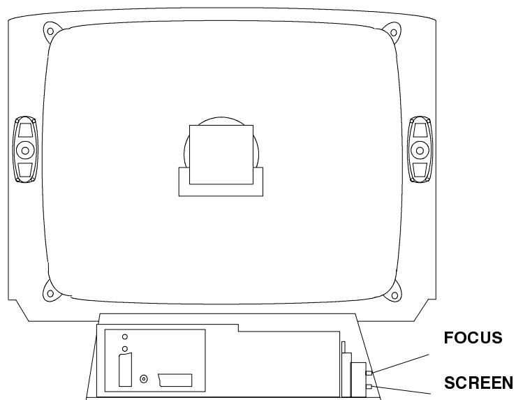
E P.C.B. Fig. 4.
